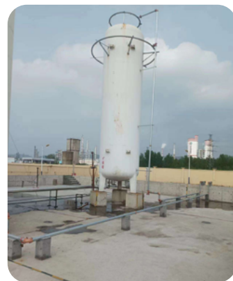
燃氣儲罐
